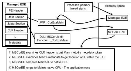
شکل (۲۵-۳) بارگذاری و مقدار دهی اولیه به CLR
