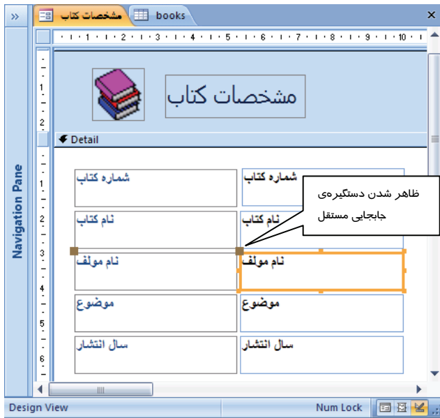
(شکل ۵-۴۱- نمای Design-انتخاب فیلد و مقدار مستقل از یکدیگر)
