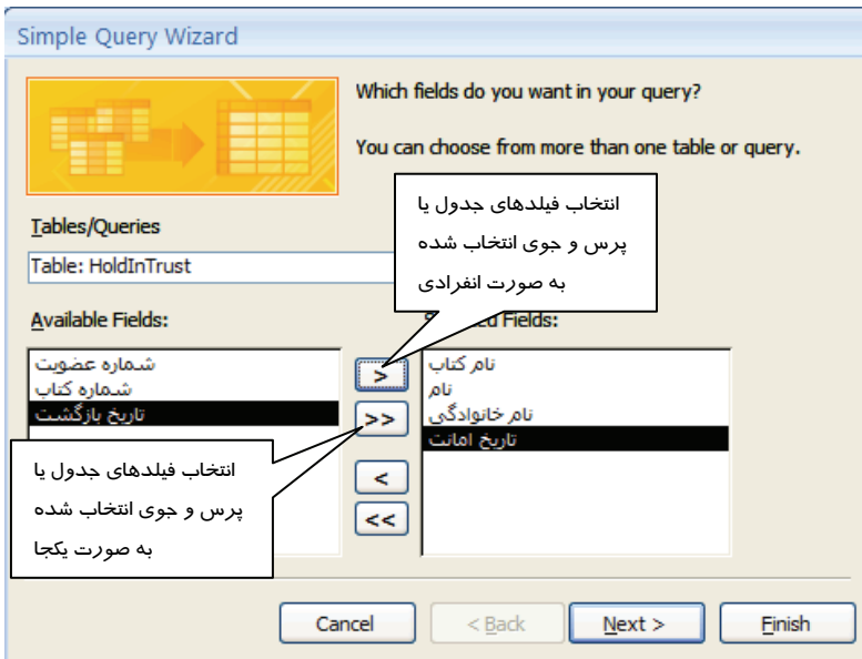
(شکل ۴-۴ دومین پنجره از Query Wizard-انتخاب فیلدها)
